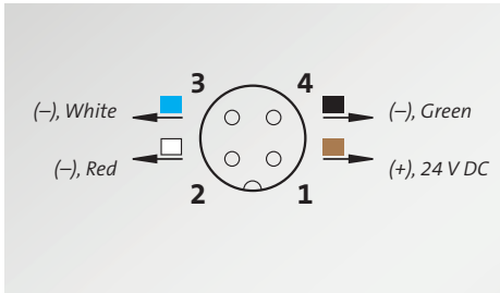
M12 connettore femmina – RGW (versione SC)
