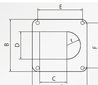
Dimensione / Dima di foratura FWS-B 29 a 48
