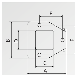
Dimensione / Dima di foratura FWS-B 11 a 21
