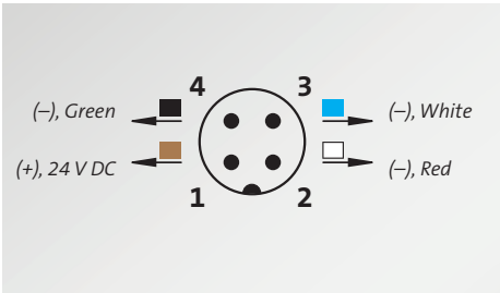
M12 connettore maschio – RGW
