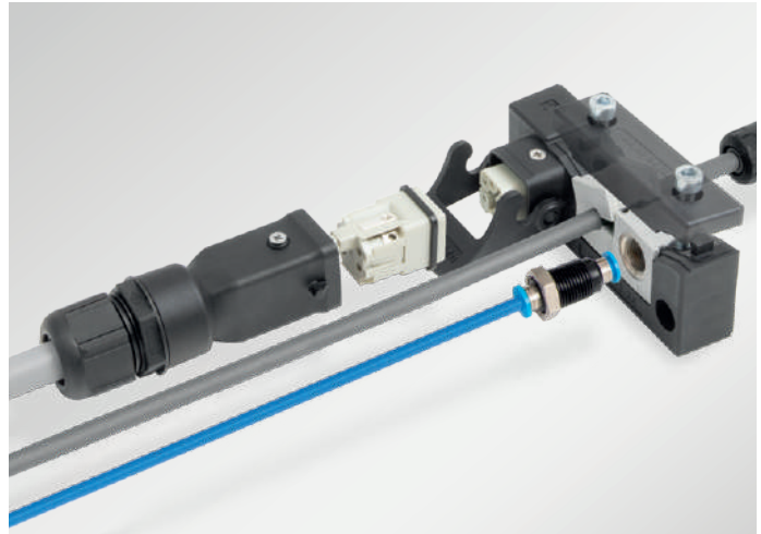
Connettore 4A e vari cavi combinati in un unico telaio
