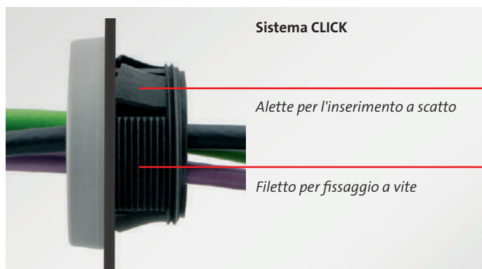
Tipo di montaggio 1: Innestrato nella foratura Per spessore parete 1 – 2,5 mm
